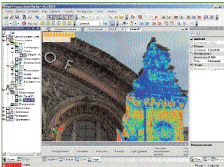
Рис. 4 Вид рабочего окна программного обеспечения Торсон ScanMaster
